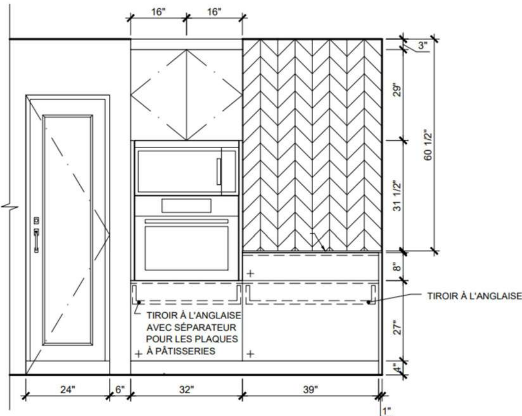
ÉLÉVATION FOUR ENCASTRÉ
