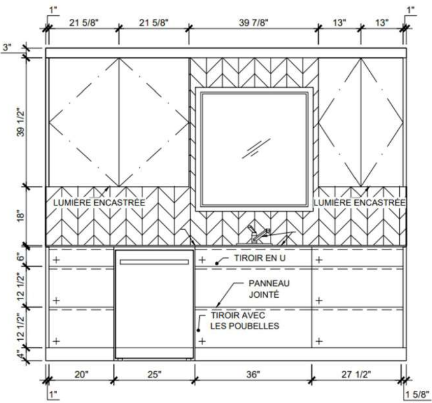
ÉLÉVATION FENÊTRE
