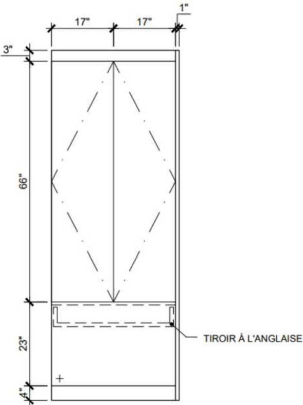
ÉLÉVATION G-M
