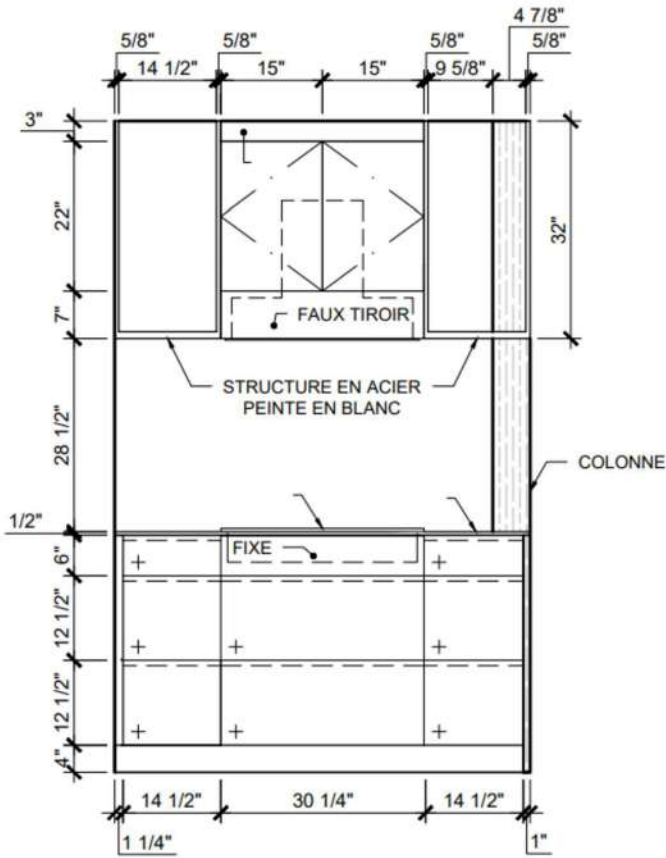
ÉLÉVATION HOTTE
