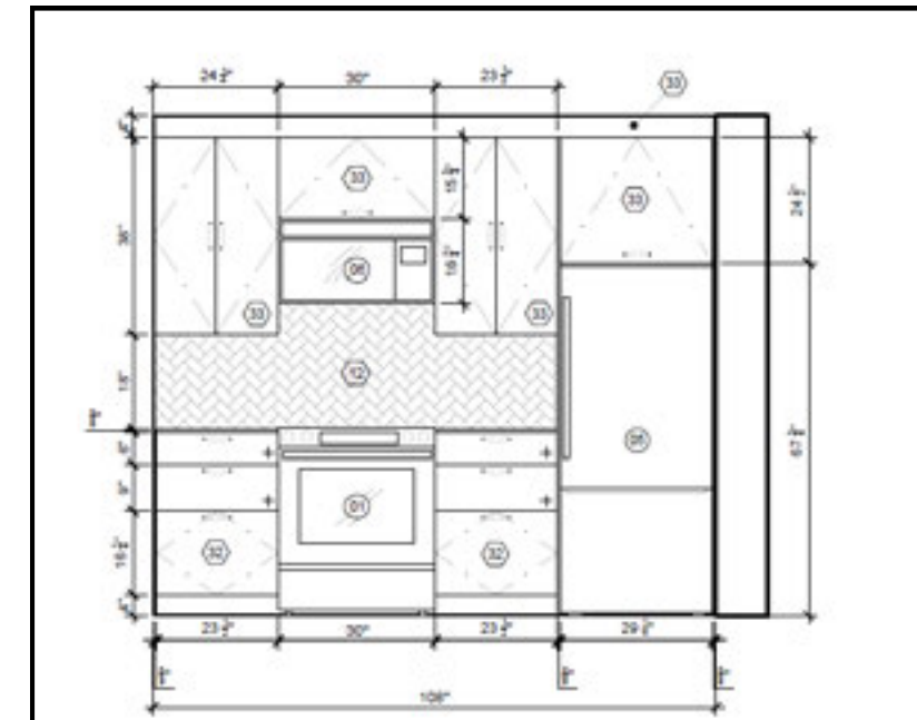
Élévation cuisine
