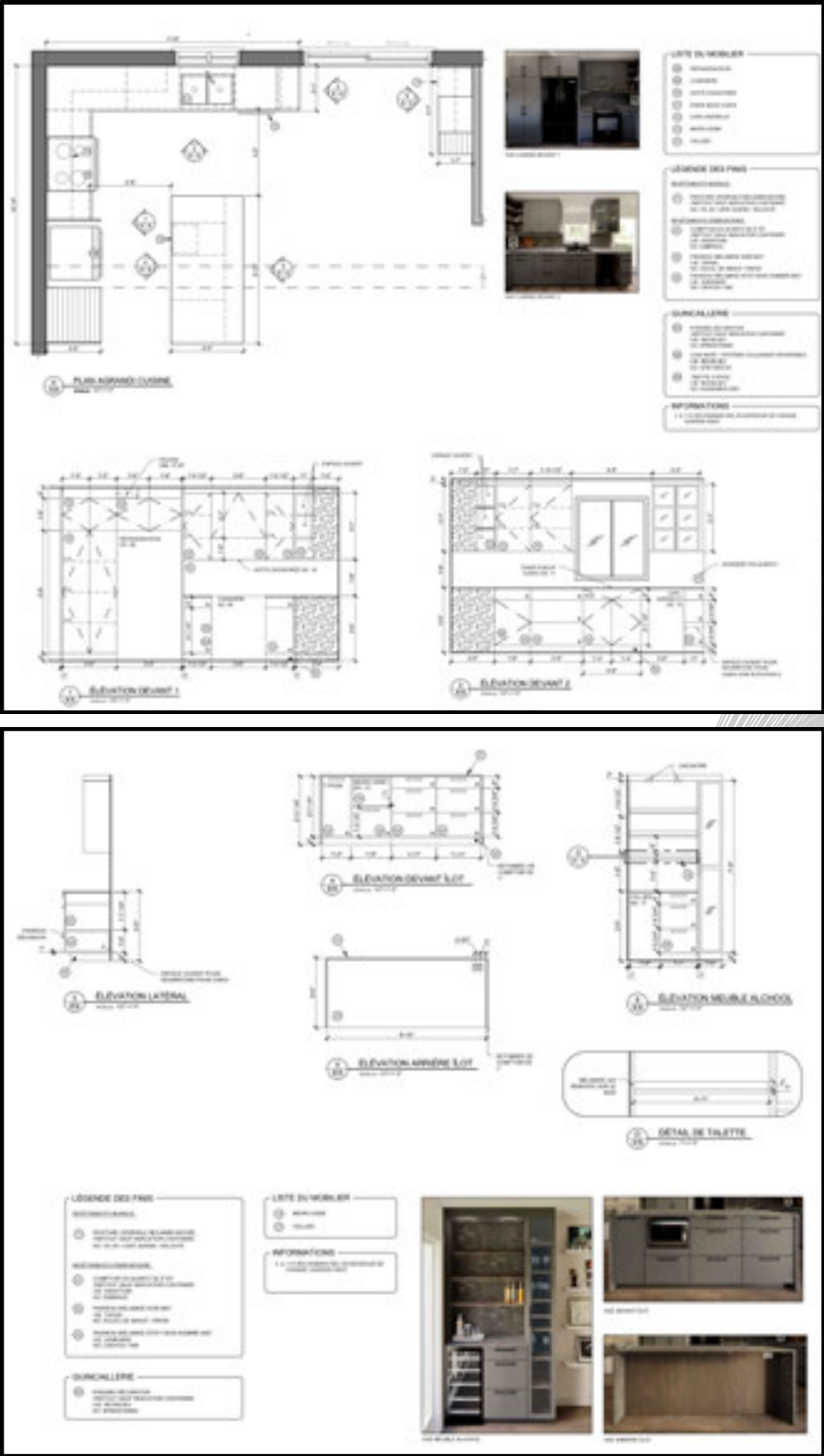
Élévations de cuisine
