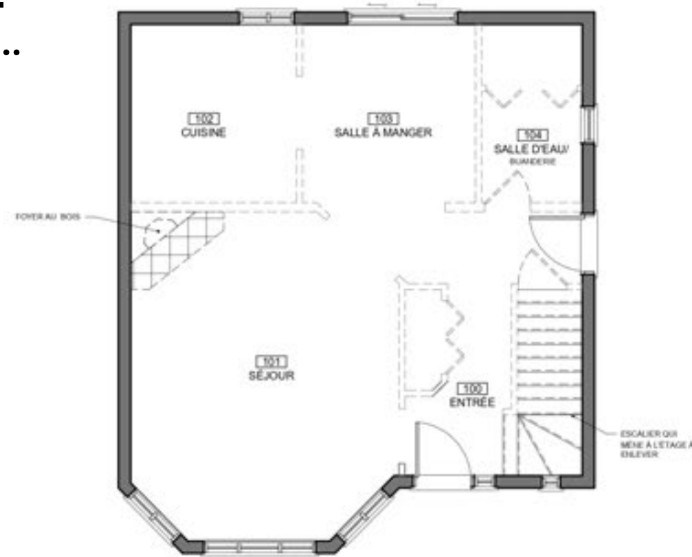
Rez-de-chaussée existant
