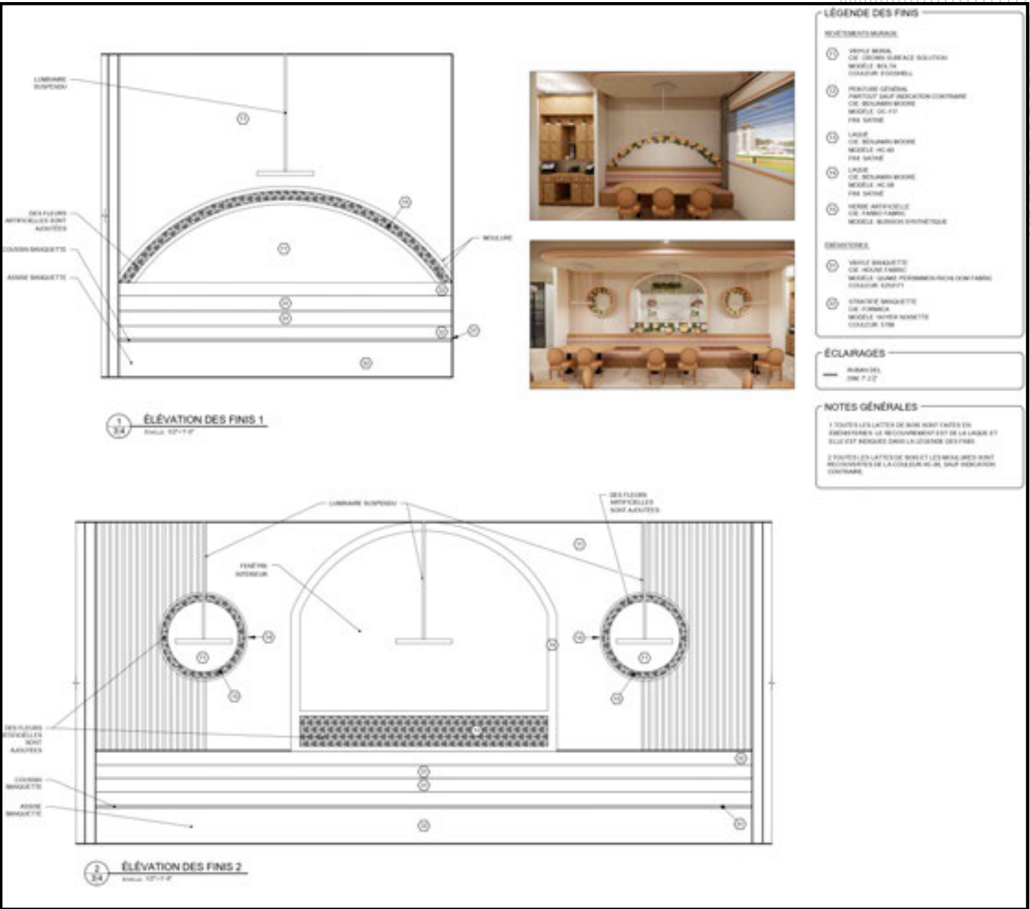
Élévations des finis
