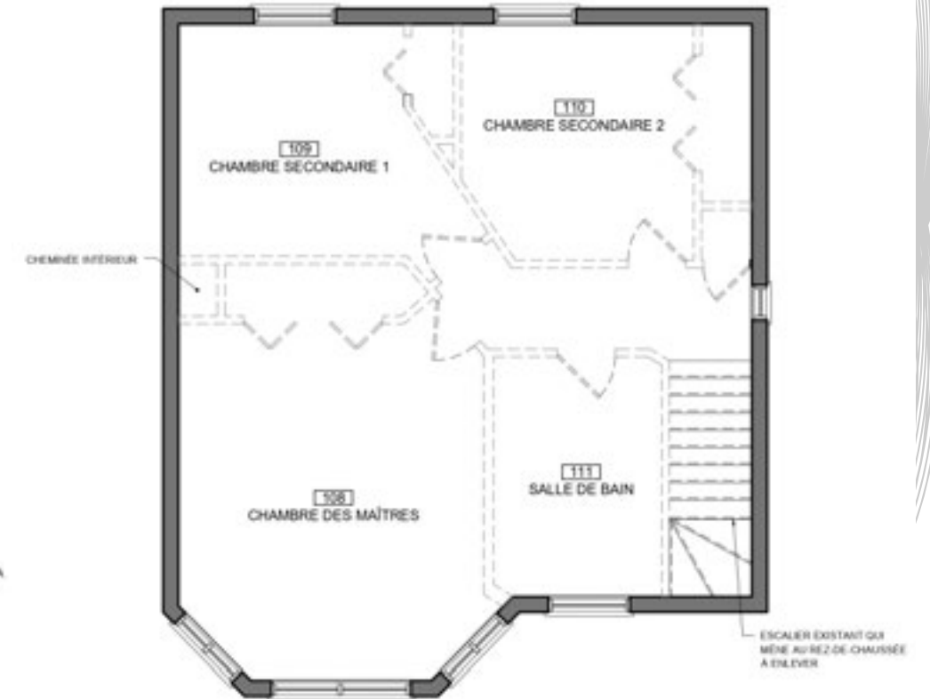
Étage existant
