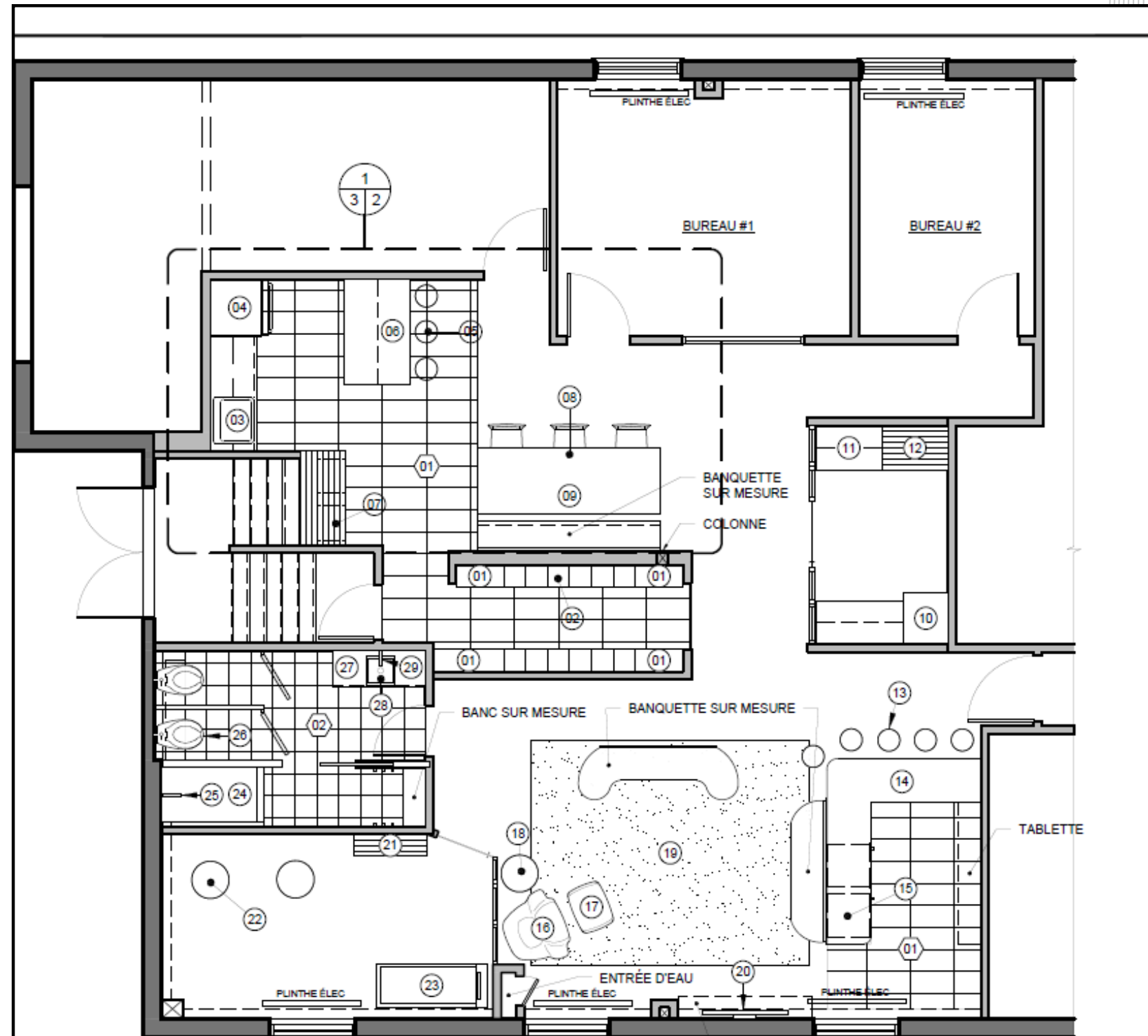
Plan d'aménagement
