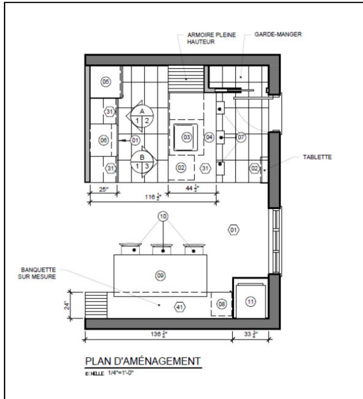
Plan d'aménagement
