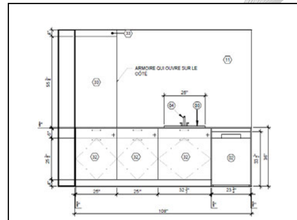
Élévation îlot
