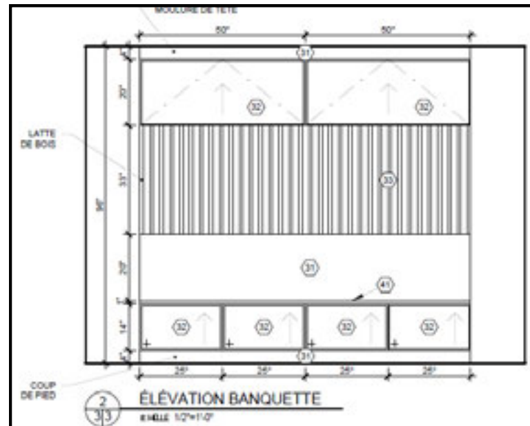
Élévation banquette
