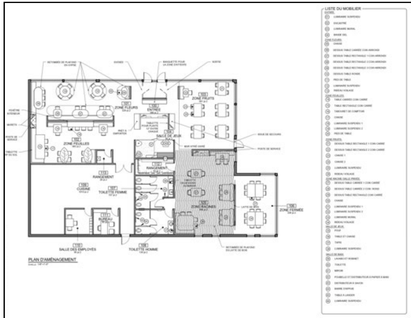
Plan d'aménagement
