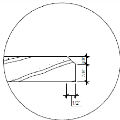
11 18/20 DÉTAIL COMPTOIR ÉCHELLE: 6"=1'-0"
