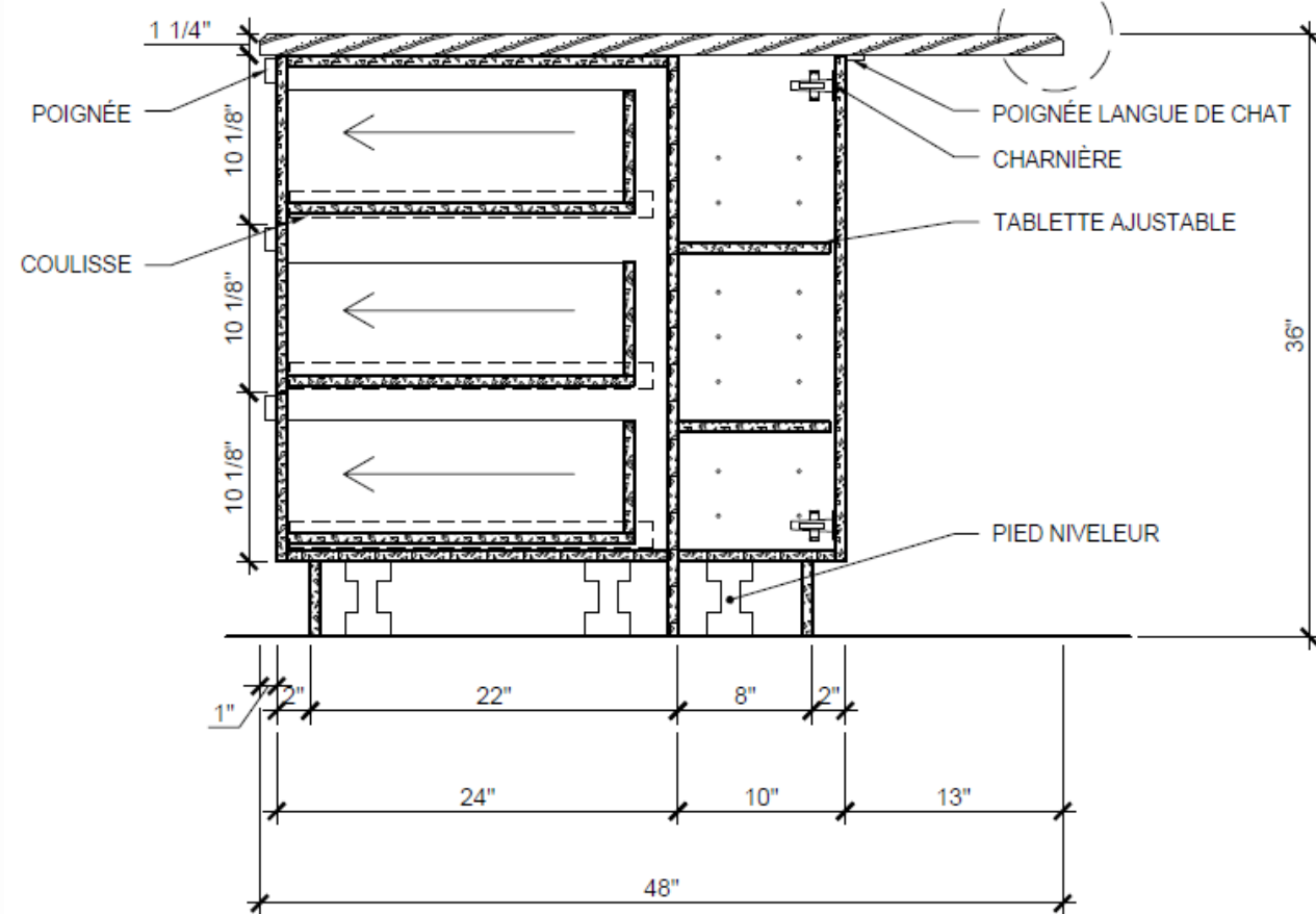
10 18/20 COUPE ÎLOT ÉCHELLE: 1"=1'-0"
