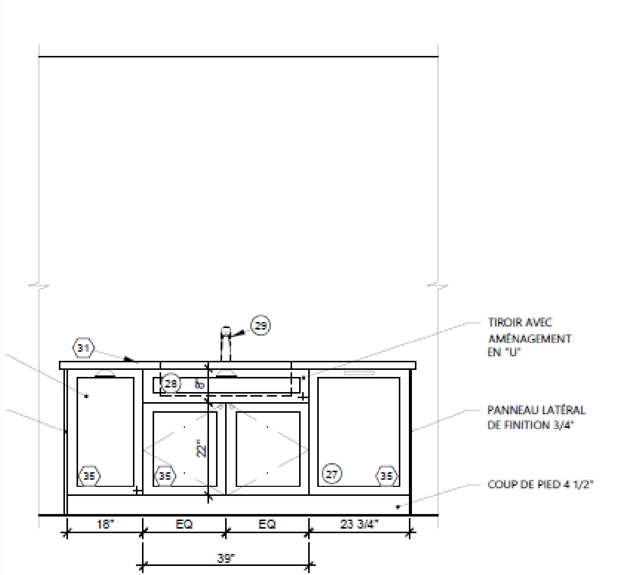
5 ÉLÉVATION CUISINE / ZONE LAVAGE Echelle: 1/2"=1'-0"
