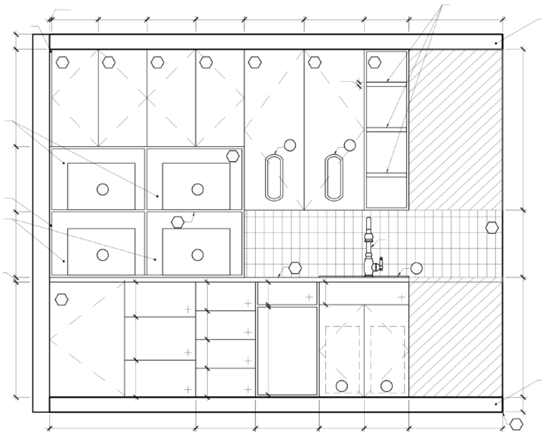
ÉLEVATION DE LA SALLE DE STÉRILISATION
