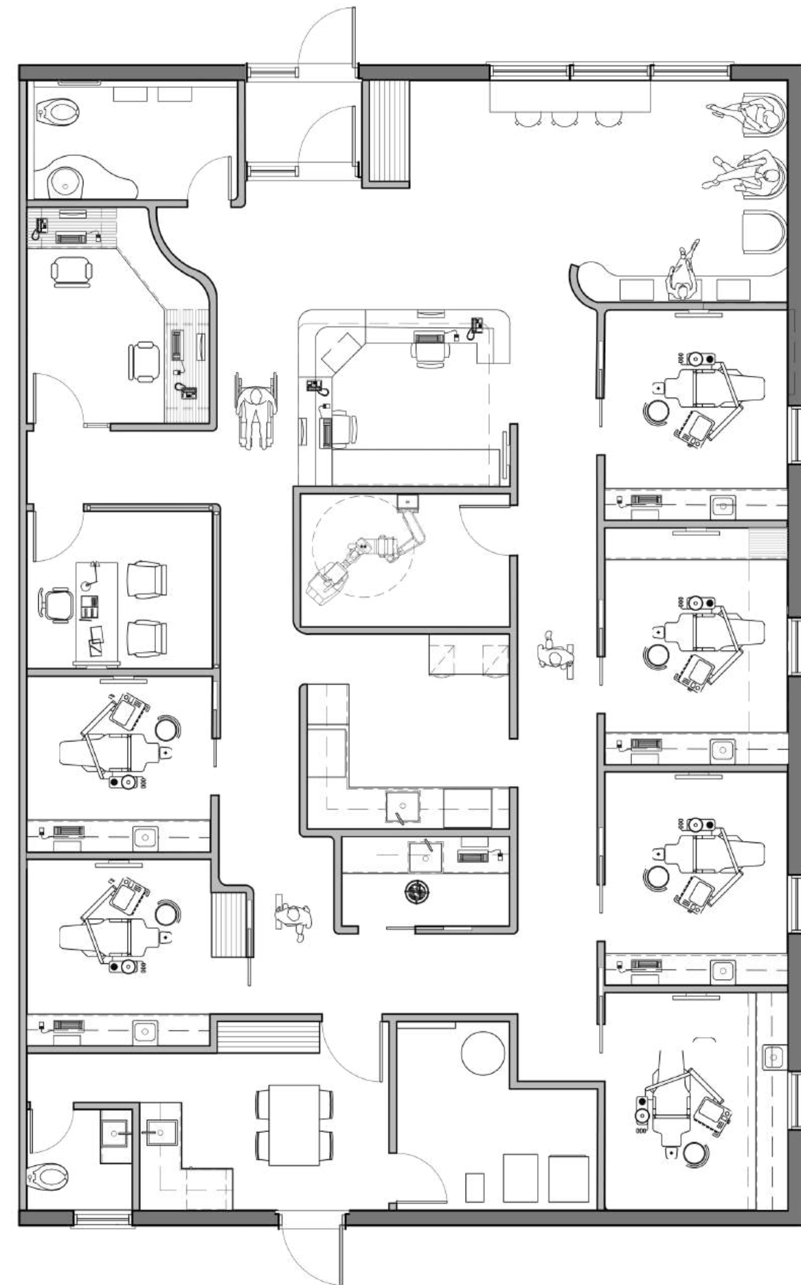
PLAN D'AMÉNAGEMENT DE LA CLINIQUE
