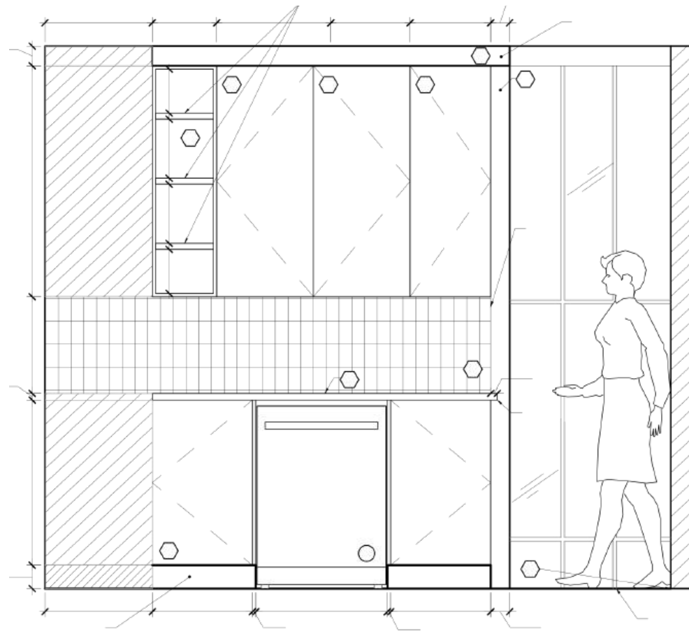
ÉLEVATION DE LA SALLE DE STÉRILISATION
