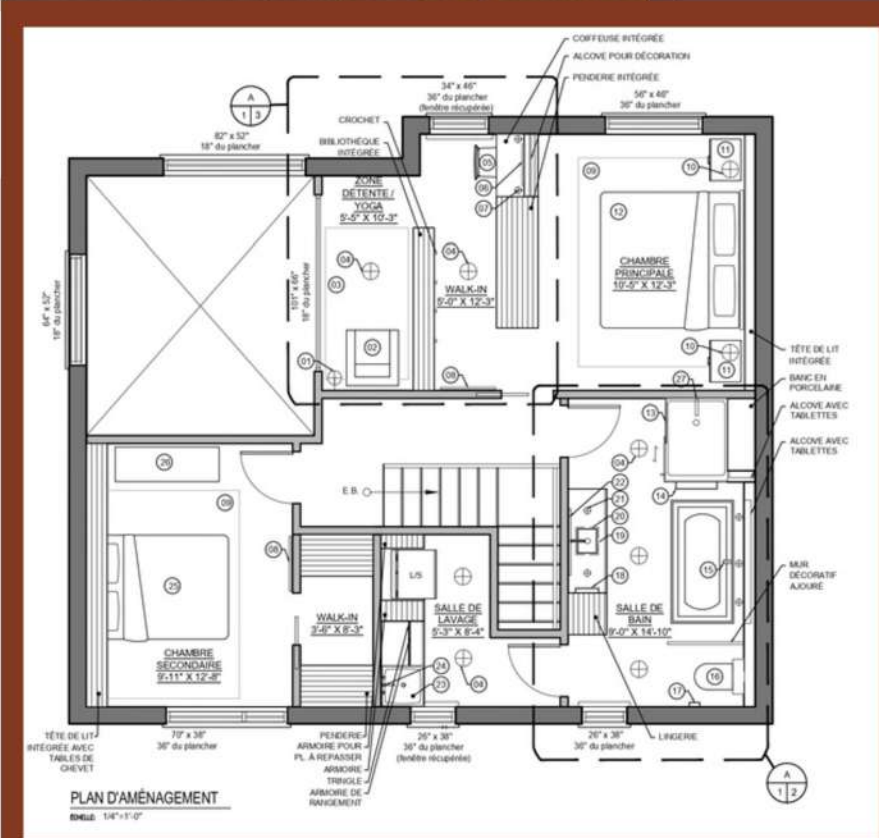
PLAN D'AMÉNAGEMENT DE L'ÉTAGE
