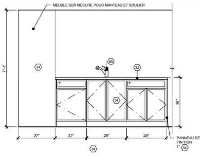
2 1/2 ÉLÉVATION ÎLOT ÉCHELLE: 1/2"=1'-0"
