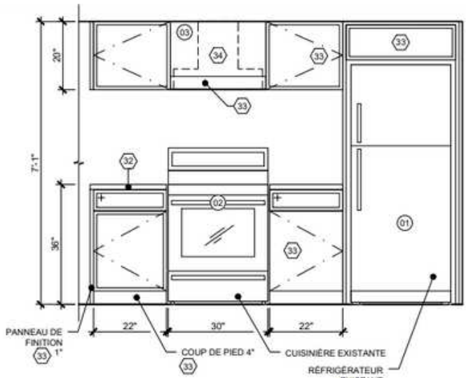
1 1/2 ÉLÉVATION DE LA CUISINIÈRE ÉCHELLE: 1/2"=1'-0"
