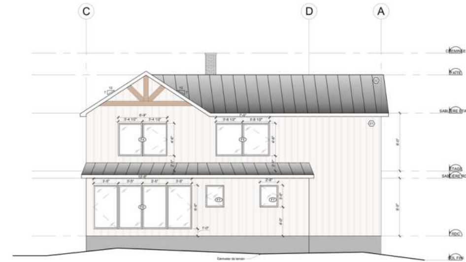
C 15 ELEVATION FAÇADE ARRIÈRE Dessiné 1/4" = 1'-0"
