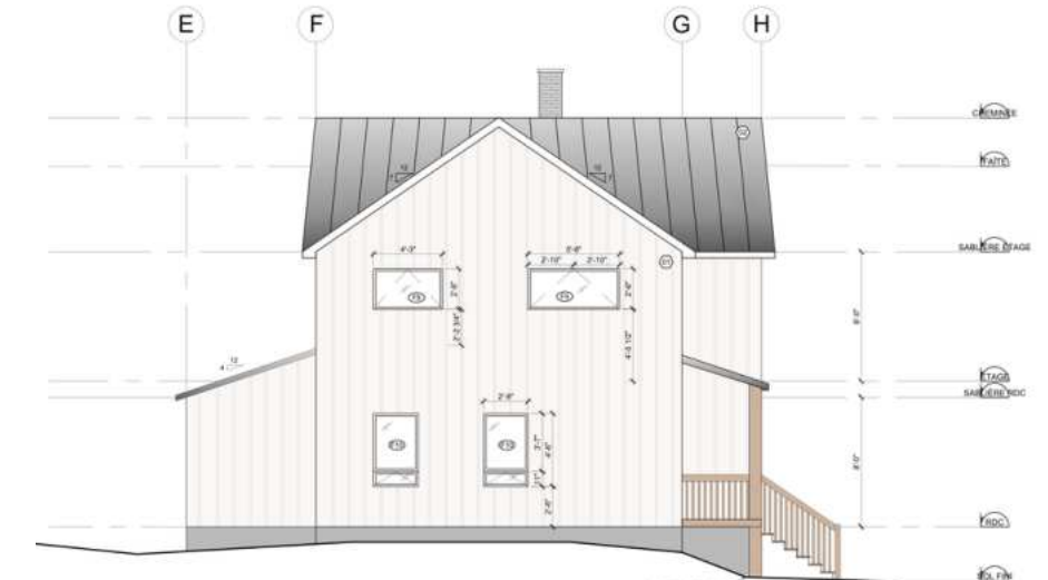
8 113 ELEVATION LATÉRALE DOWLE 11/11/14
