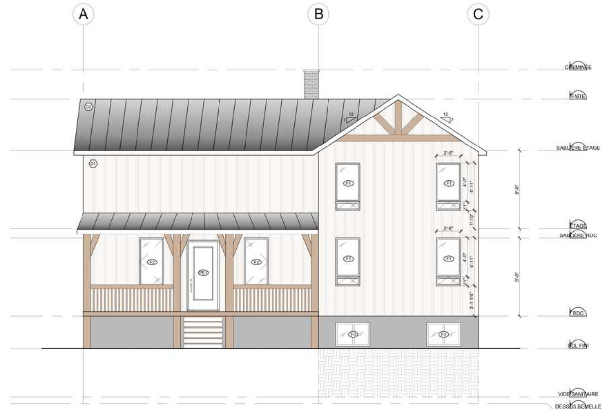
ELEVATION FAÇADE AVANT Echelle: 1/4"=1'-0"
