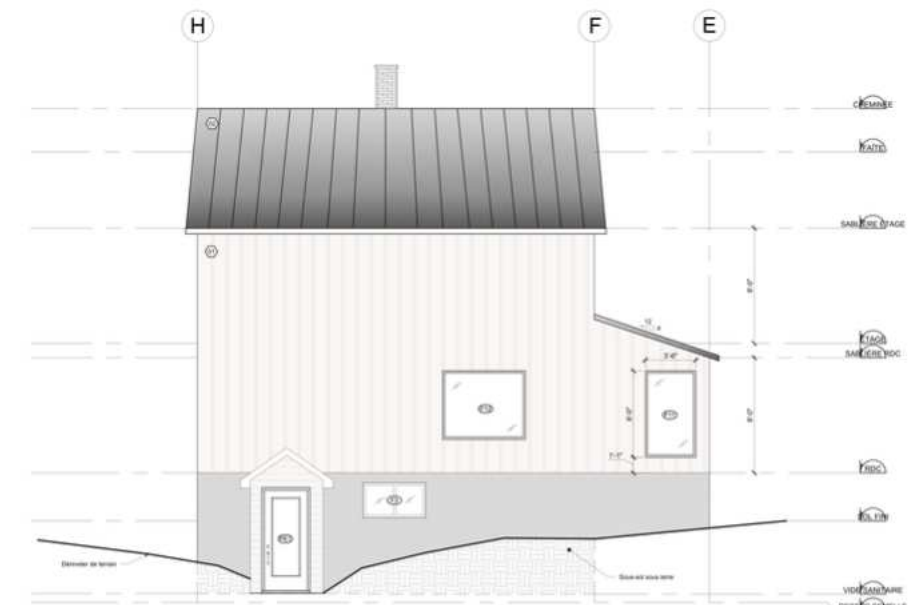
0 16 ELEVATION LATÉRALE Châssis: 147x112"
