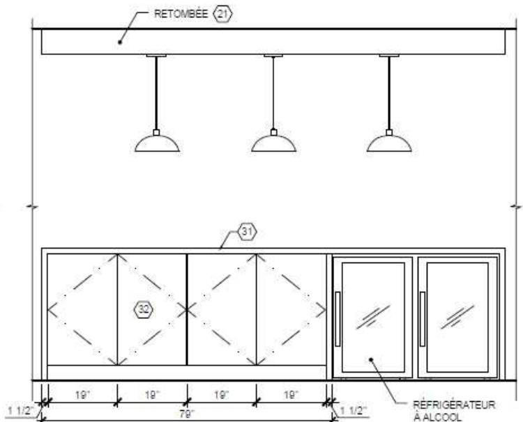
3 3/4 ÉLEVATION ÎLOT DU BAR ÉCHELLE: 1/2"=1'-0"
