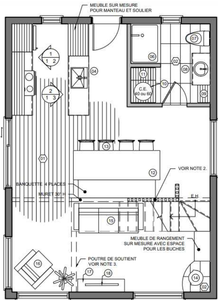
PLAN D'AMÉNAGEMENT ÉCHELLE: 1/4"=1'-0"
