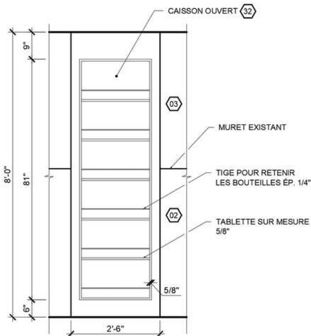
4 3/5 ÉLEVATION COMPTOIR LUNCH ÉCHELLE: 1/2"=1'-0"
