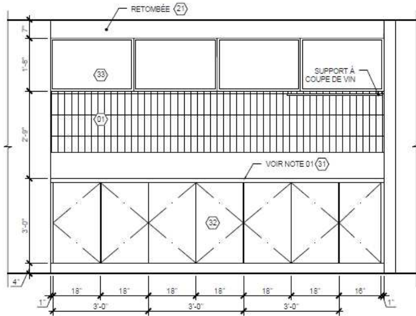
2 3/4 ÉLEVATION DU BAR ÉCHELLE: 1/2"=1'-0"
