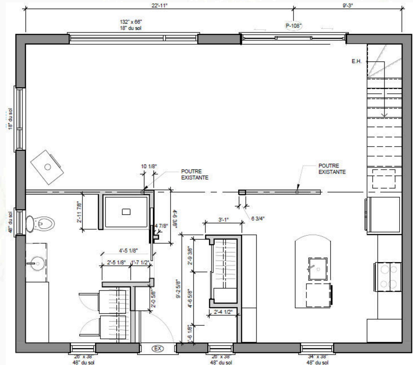
Plan de construction
