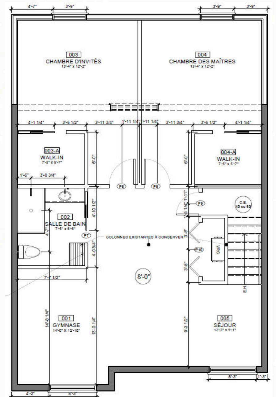
Plan de démolition / construction
