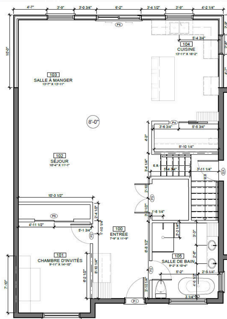
Plan de construction
