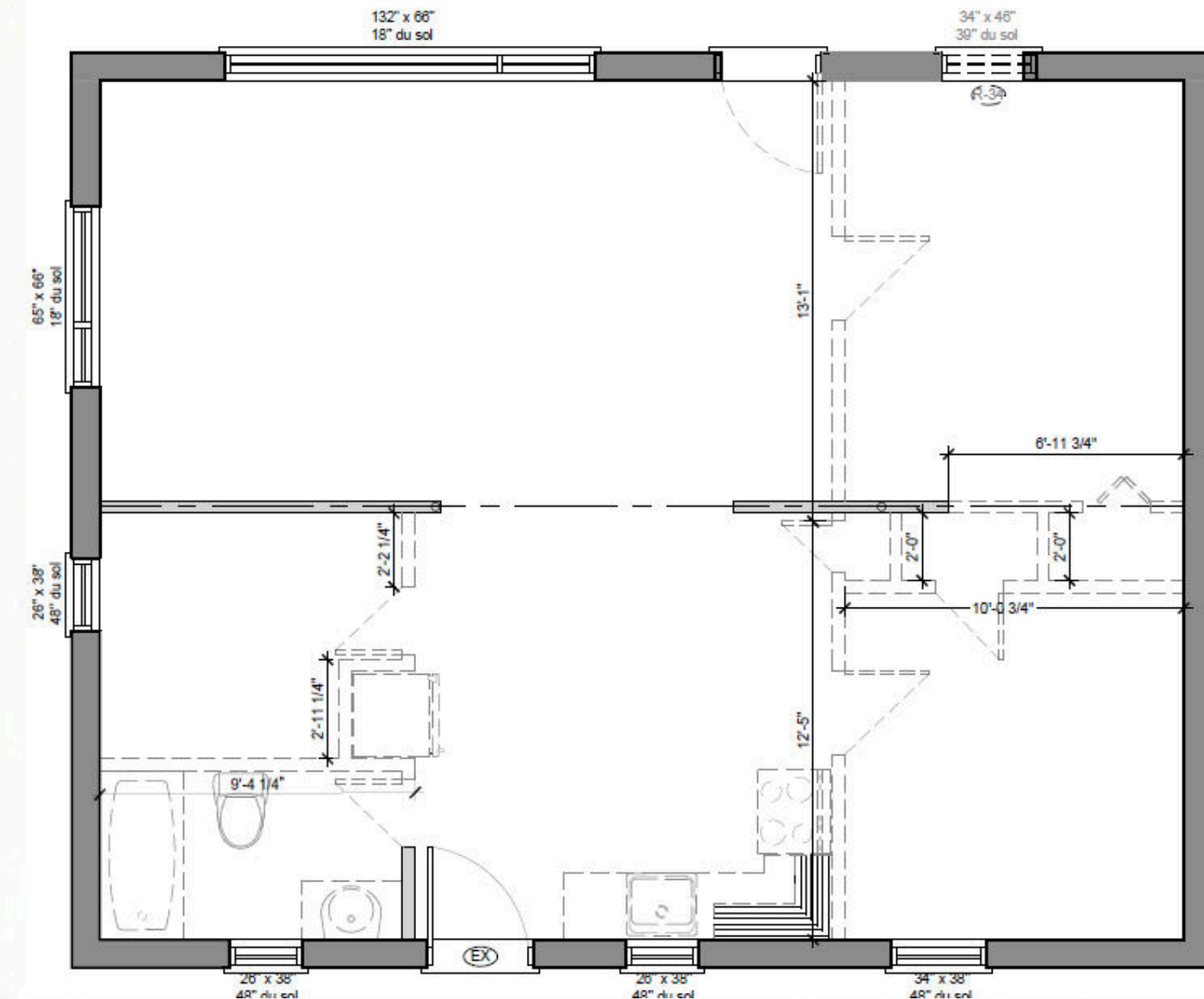
Plan de démolition
